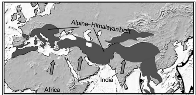
Рис. 4. Обзорная карта Альпийско-Гималайского складчатого пояса.
